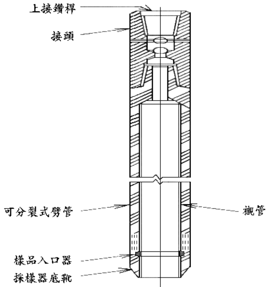
圖三 劈管採樣器
