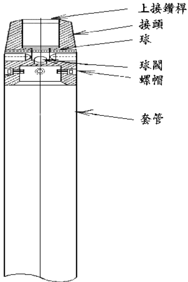
圖四 薄管採樣器
