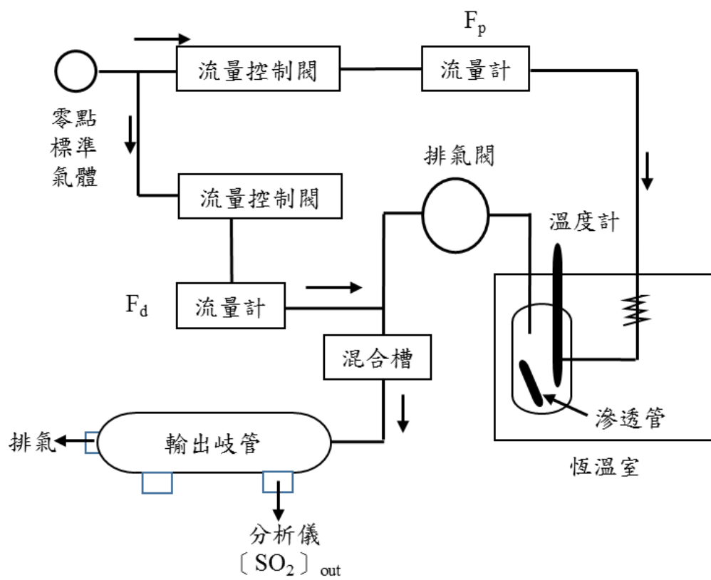
圖三、滲透管法之校正系統示意圖
