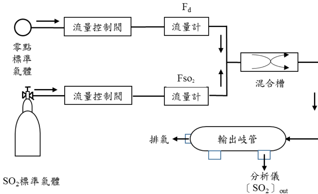
圖一、二氧化硫自動分析儀器示意圖
