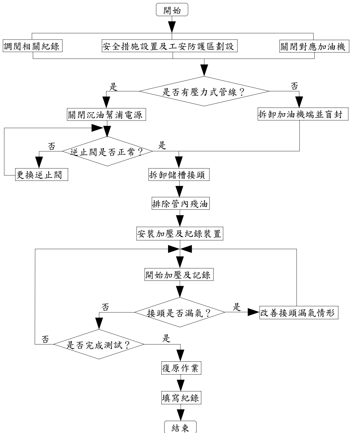
圖一 儲槽系統管線密閉測試作業流程
