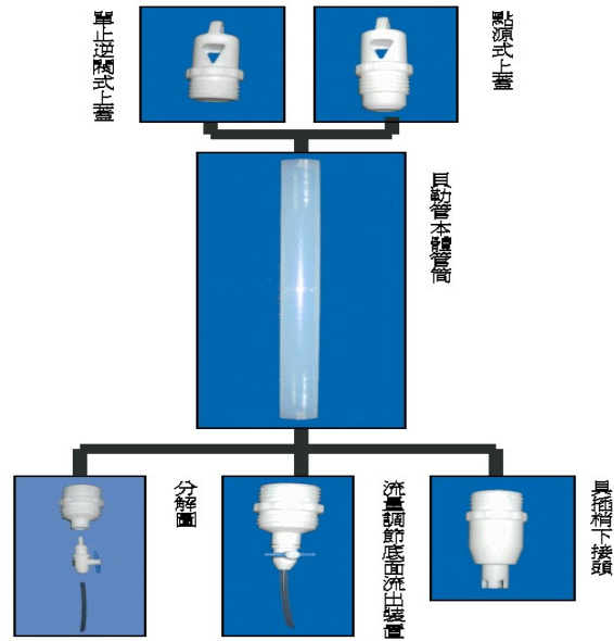
圖一 貝勒管及其配件
